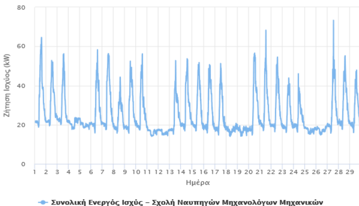
Εικόνα 14: Συνολική ζήτηση ισχύος για το μήνα αναφοράς - Σχολή Ναυπηγών Μηχανολόγων Μηχανικών
