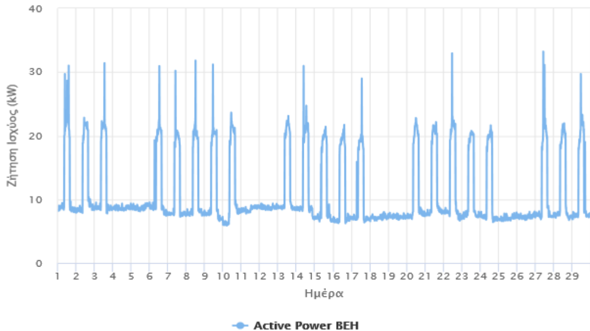
Εικόνα 6: Συνολική ζήτηση ισχύος για το μήνα αναφοράς - Σχολή Αγρονόμων και Τοπογράφων Μηχανικών
