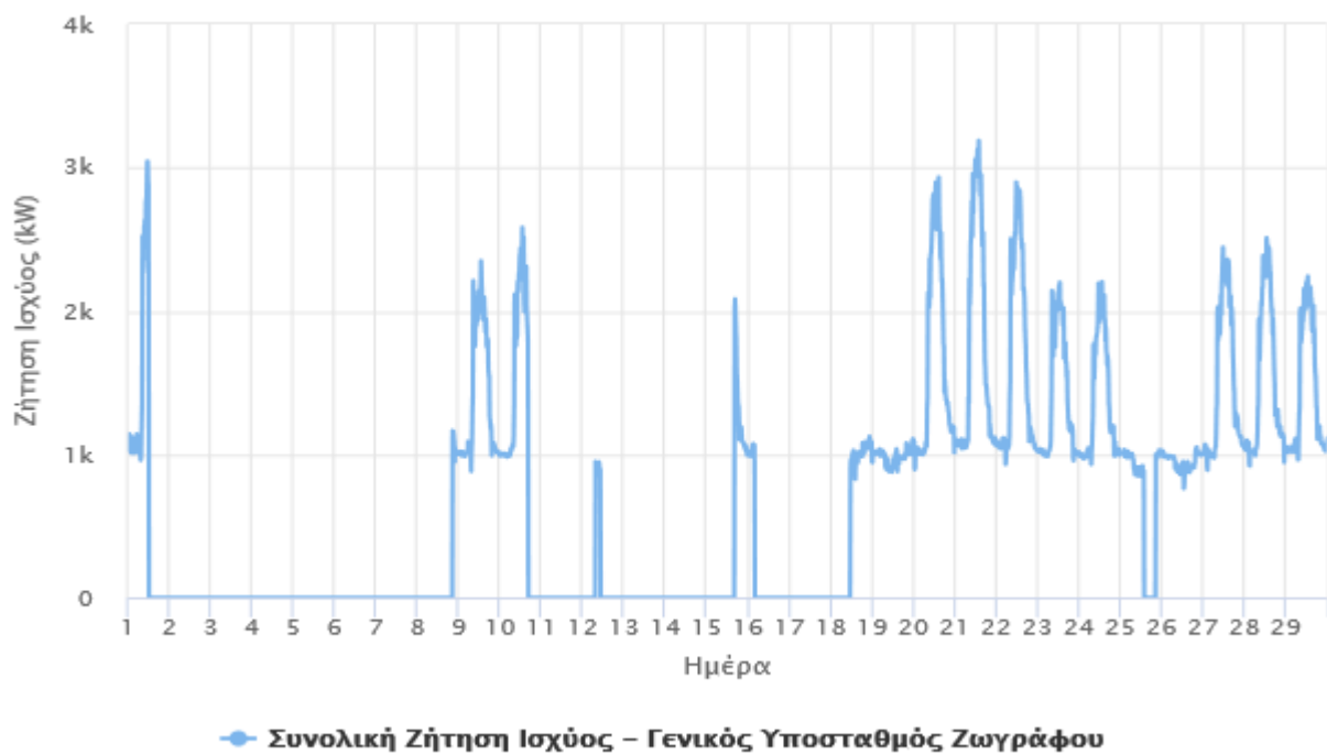
Εικόνα 1: Συνολική ημερήσια ζήτηση ισχύος για τον εξεταζόμενο μήνα
