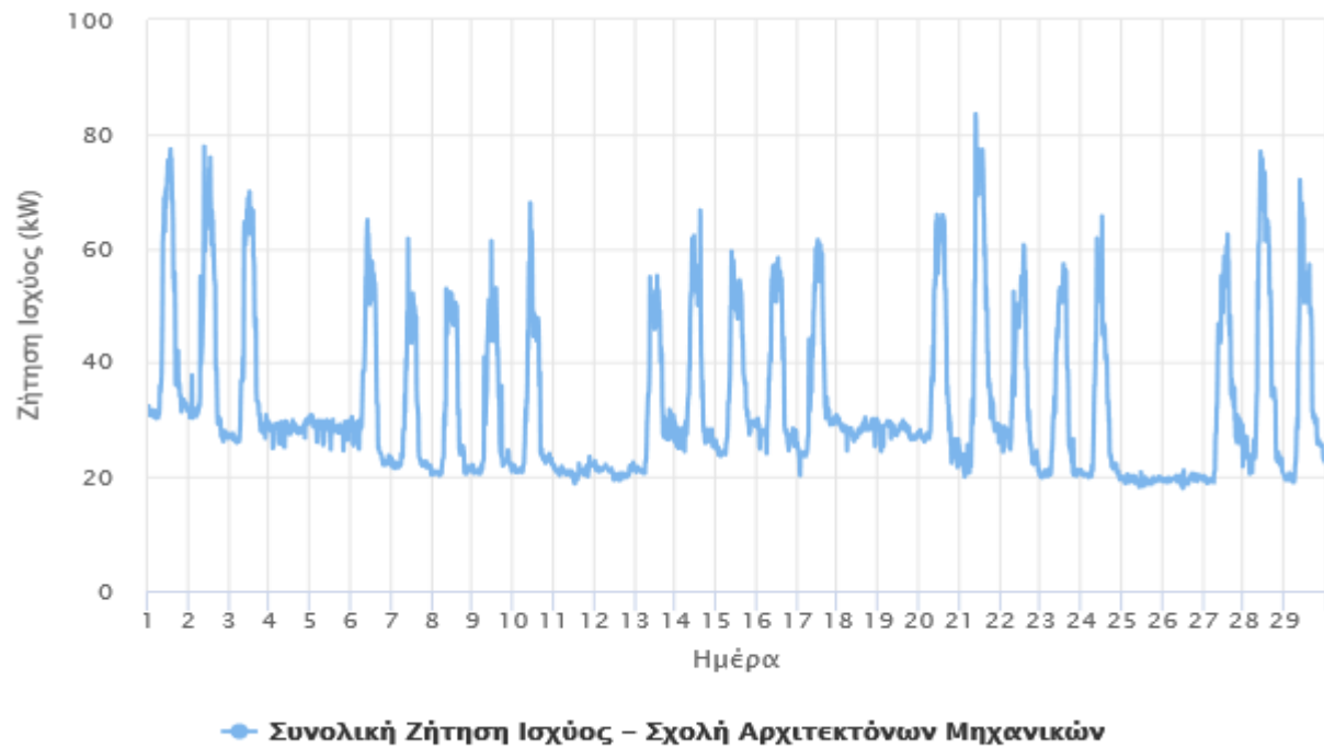
Εικόνα 17: Συνολική ζήτηση ισχύος για το μήνα αναφοράς - Σχολή Αρχιτεκτόνων Μηχανικών
