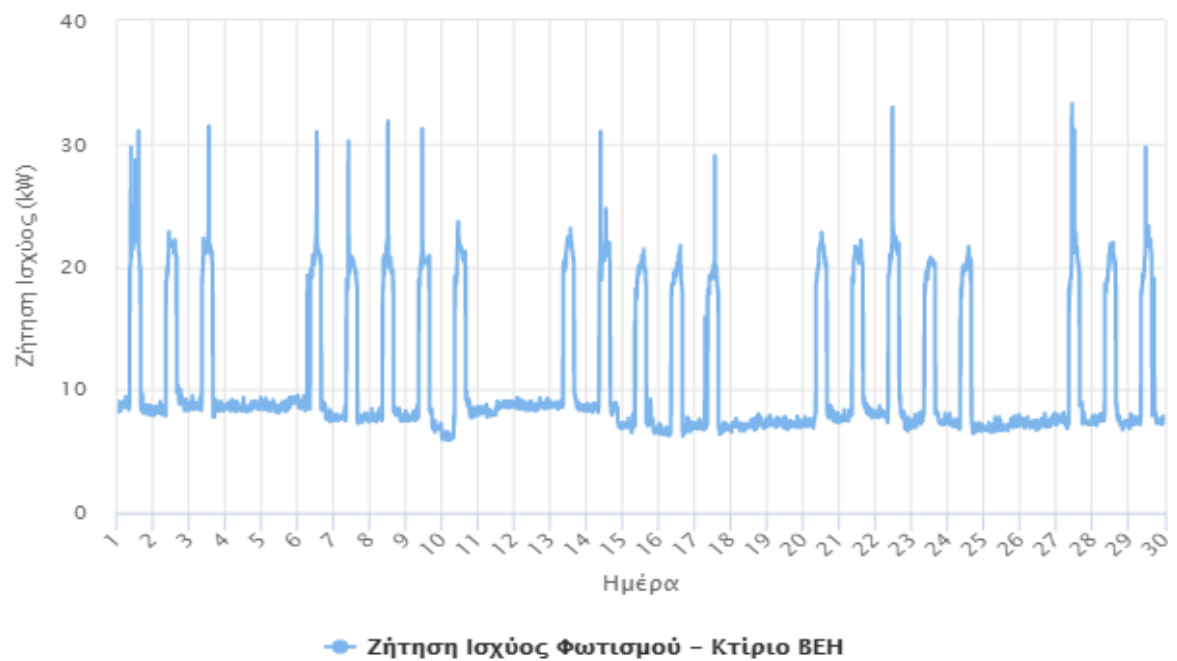
Εικόνα 7: Συνολική ζήτηση ισχύος φωτισμού για το μήνα αναφοράς - Κτίριο ΒΕΗ
